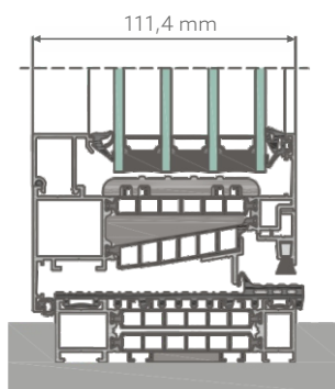
KRYŽMINIS SKIRSNIS SU ŽEMA PALANGE TM 102HI
