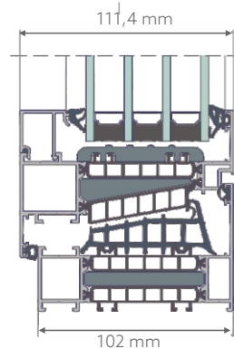
KRYŽMINIS SKIRSNIS LANGO TM 102HI
