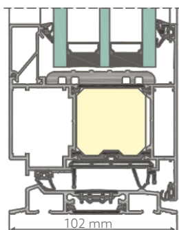
KRYŽMINIS SKIRSNIS DURŲ VARTŲ
